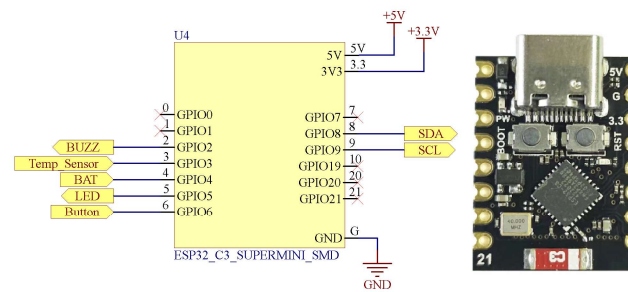
Microcontroller(ESP32 C3 Super-mini)
